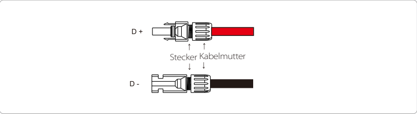
Schematische Darstellung des angeschlossenen PV-Wechselrichters.
