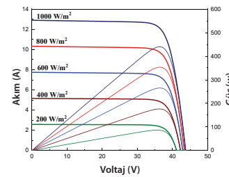
Akım - Voltaj &amp; Güç - Voltaj Grafiği(46PMSHFB)
