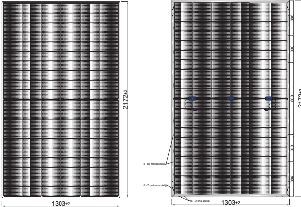
ÖNDEN GÖRÜNÜM
