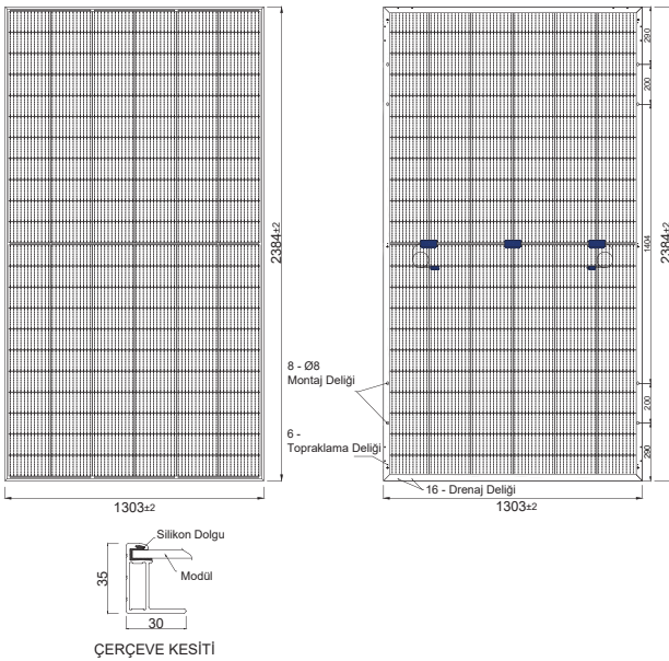
ÖN GÖRÜNÜŞ
