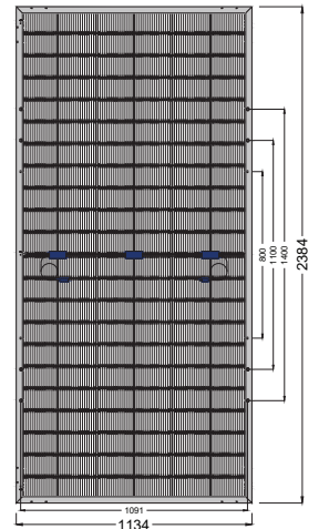
ARKADAN GÖRÜNÜM
