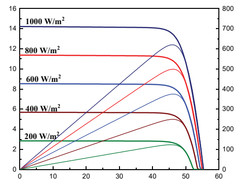
Strom - Spannungs & Leistung - Spannungs Kurve (TT620-156TN10)
