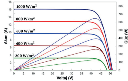
Akım - Voltaj & Güç - Voltaj Grafiği (CWT645 - 198TNBTS12R)
