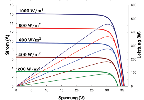
Strom-Spannungs & Leistung-Spannungs Kurve (TT455-96TNB12R)
