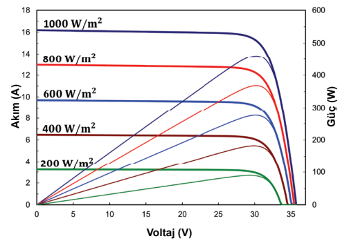
Akım - Voltaj &amp; Güç - Voltaj Grafiği (TT455-96TNB12R)
